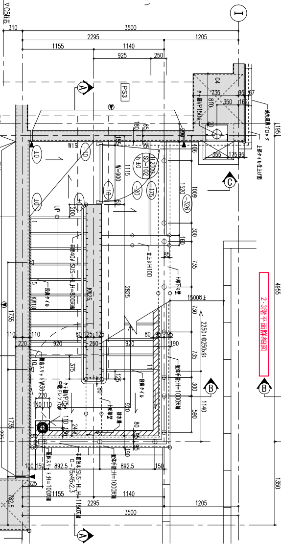
3階平面詳細図
