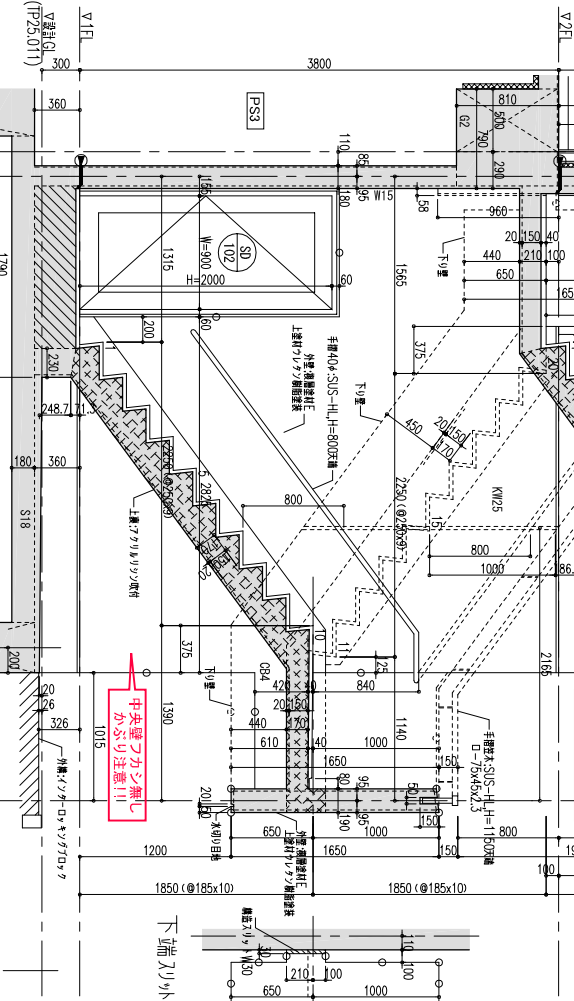
6階平面詳細図
